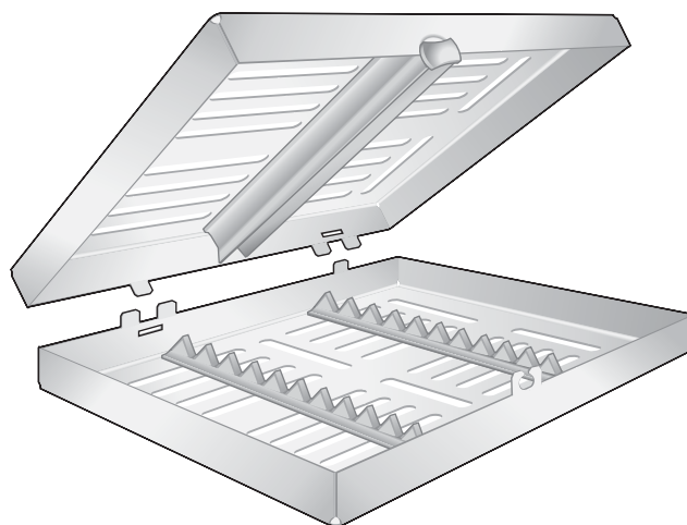
BS-60 Für 10 Instrumente For 10 Instruments Per 10 strumenti Para 10 instrumentos Pour 10 instruments 185 x 135 x 35 mm
