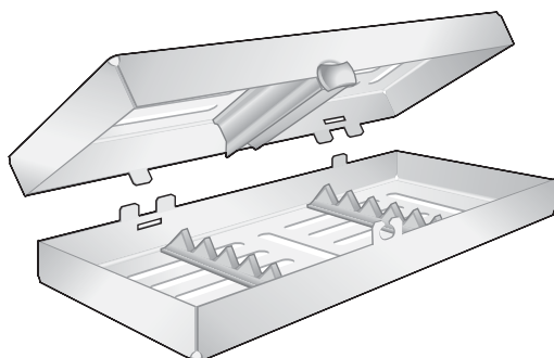
BS-59 Für 5 Instrumente For 5 Instruments Per 5 strumenti Para 5 instrumentos Pour 5 instruments 185 x 75 x 35 mm
